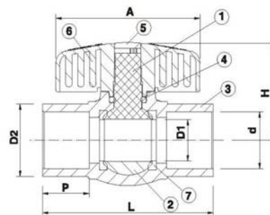
DN15~DN50
